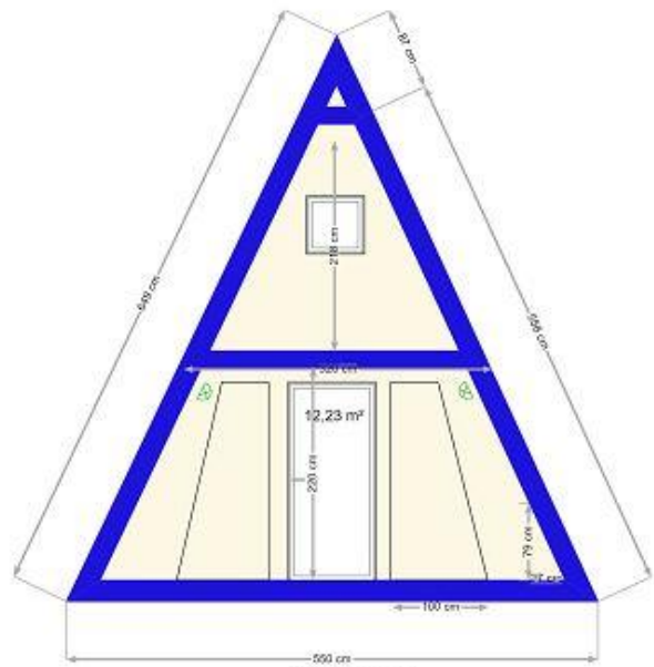
Façade sud
