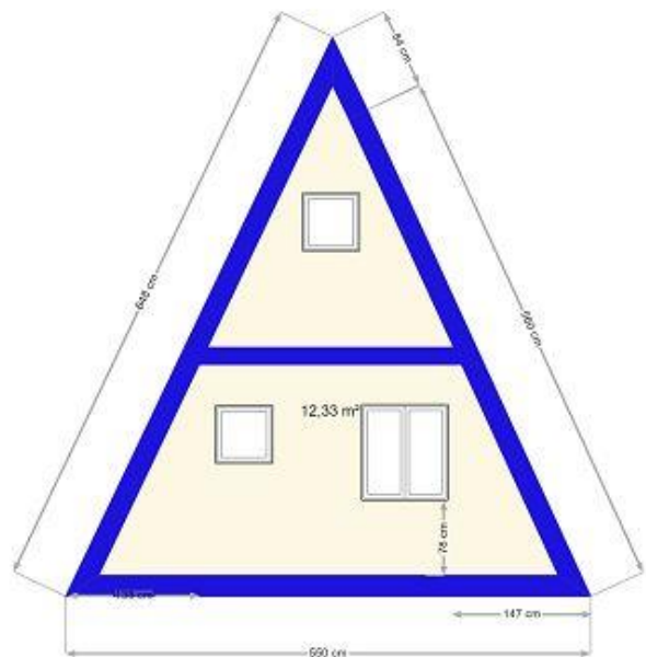
Façade nord
